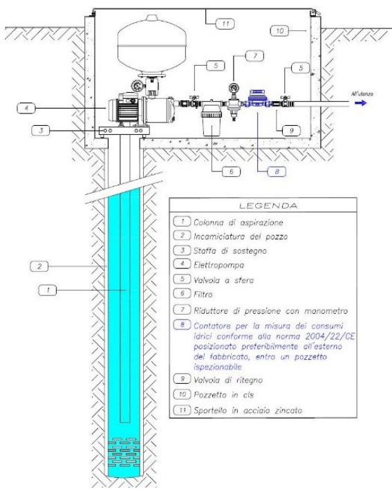
SCHEMA IMPIANTO CON APPROVV. DA POZZO
